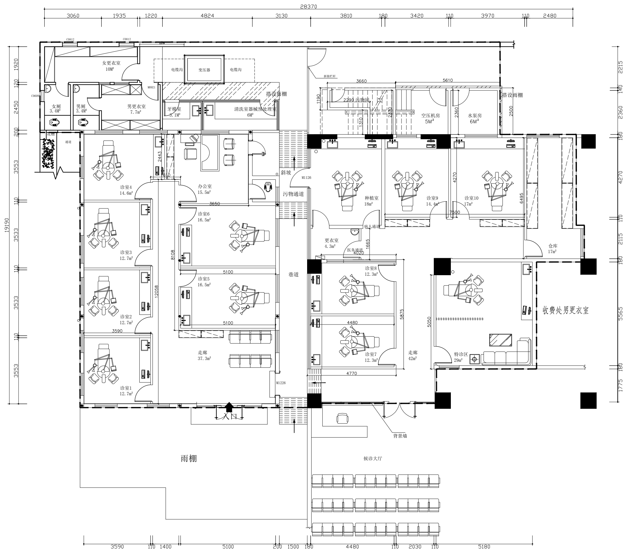
改造后平面方案图
